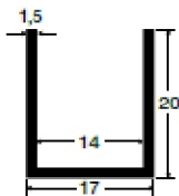
20x17x20x1,5
