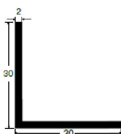
30x30x2
