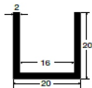
20x20x20x2
