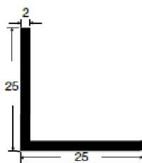
25x25x2
