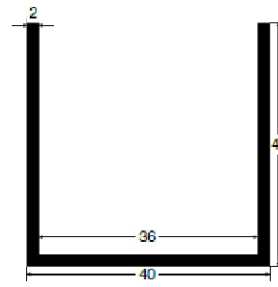
40x40x40x2
