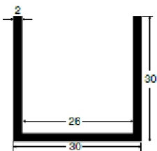
30x30x30x2
