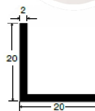
20x20x2
