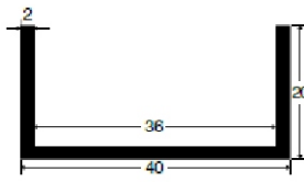
20x40x20x2
