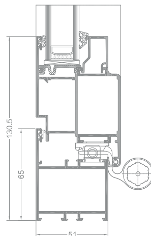
řez dveřmi EL 011 + EL 022
