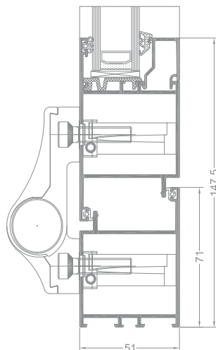
řez dveřmi EL 014 + EL 025
