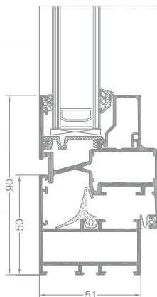
řez oknem EL 010 + VL 820
